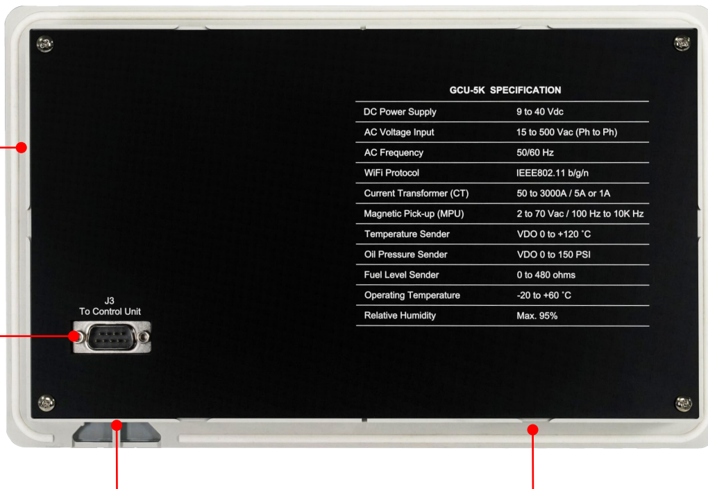
背面図
